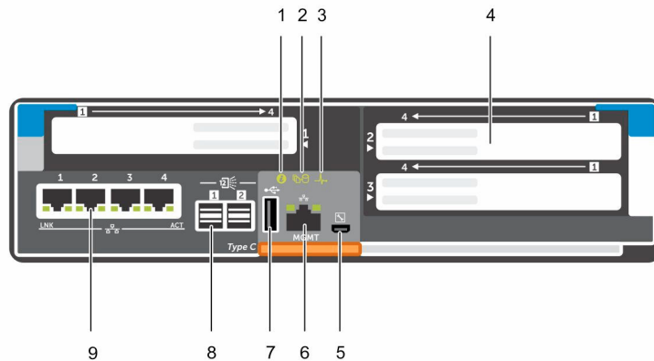
Abbildung 5. SC7020-Speicher-Controller
