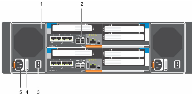
Abbildung 2. Speichersystem SC7020 Ansicht der Rückseite
